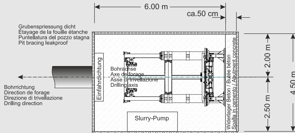
Grundriss / Coupe horizontale / Proiezione orizzontale / Top view
