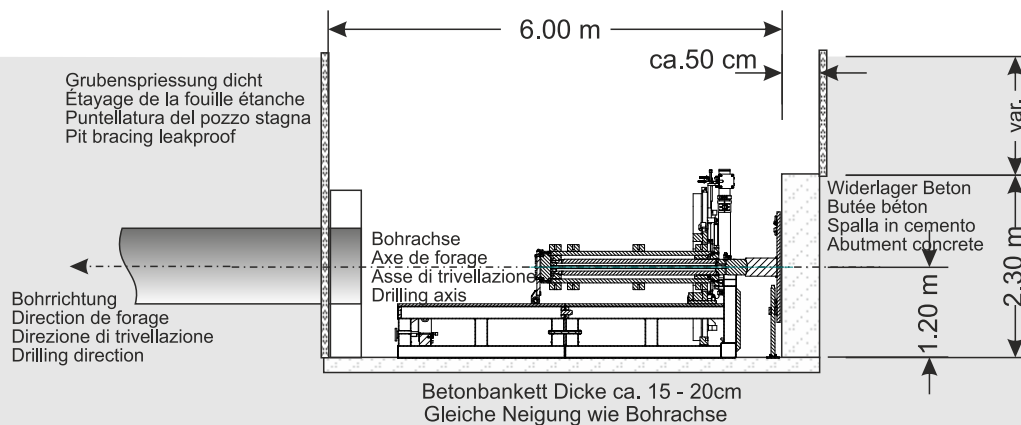
Schnitt / Coupe verticale / Proiezione verticale / Side view
